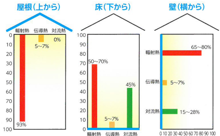
建物内を移動する熱の割合
